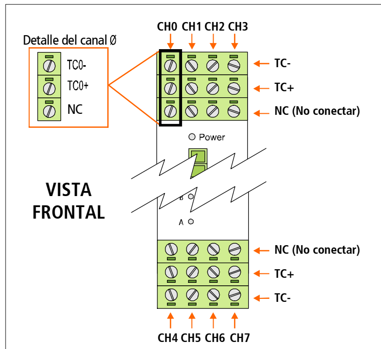
Figura 11 – Disposición de las entradas analógicas en cada canal del adquisidor RMS1-TC.
