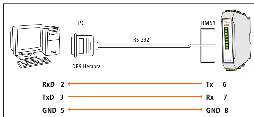
Figura 8 – Cable de conexión serie RS232 para la comunicación con una PC
