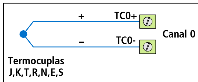
Figura 12 – Conexión de una Termocupla.
