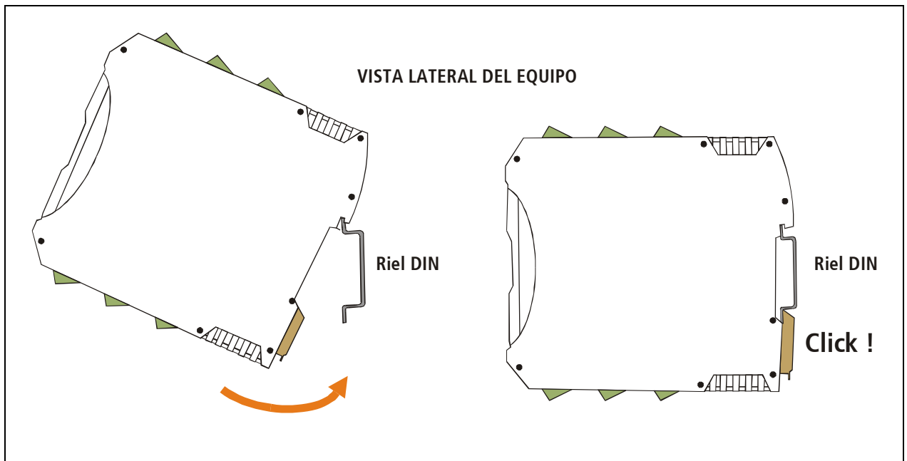
Figura 14 – Montaje del equipo
