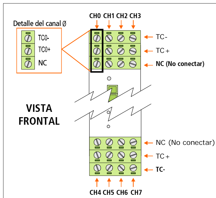
Figura 10 – Disposición de las entradas analógicas en cada canal del adquisidor RME1-TC
