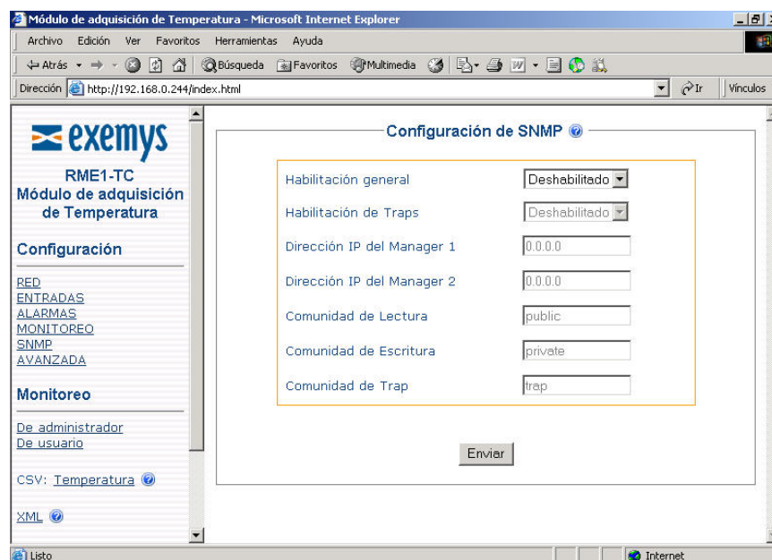
Figura 23 – Configuración de SNMP
