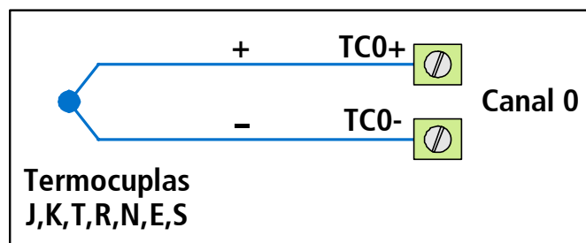
Figura 11 – Conexión de una Termocupla.
