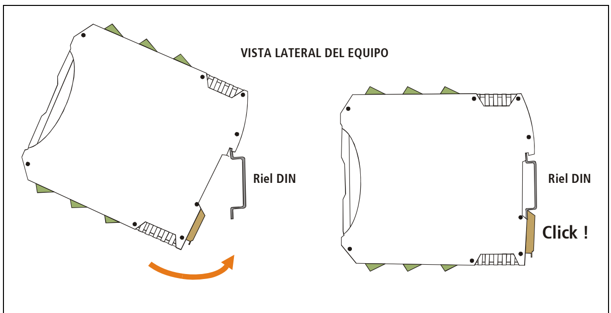
Figura 27 – Montaje del equipo
