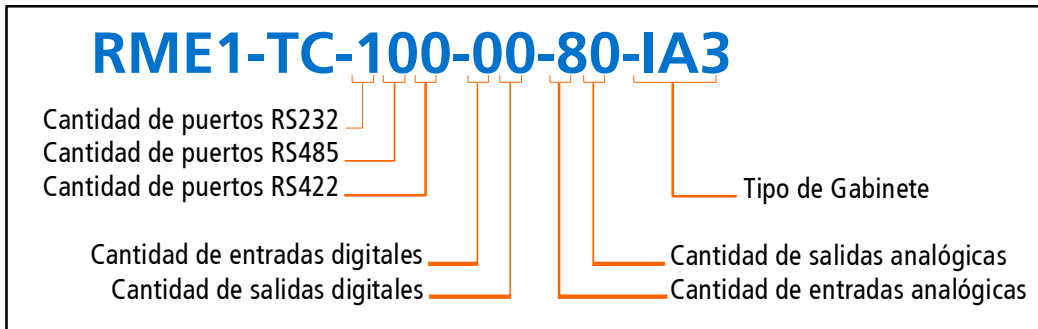
Figura 2 – Detalle de codificación de modelos
