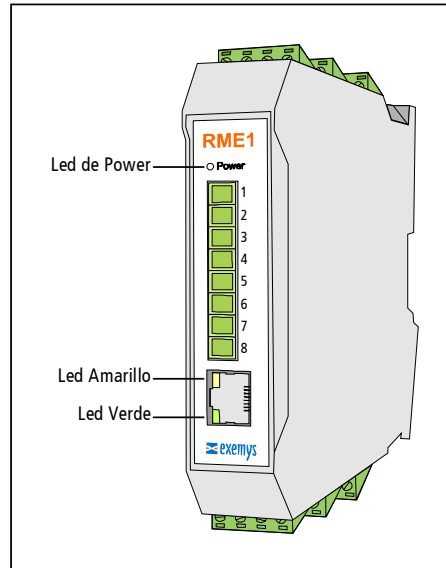
Figura 13 – Leds Indicadores
