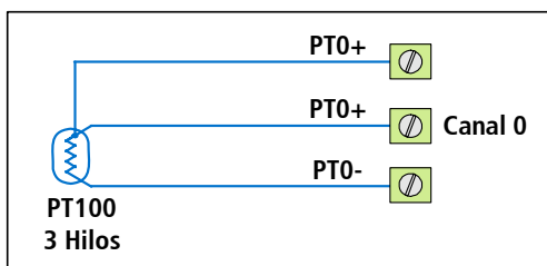
Figura 11 – Conexión PT100 3 Hilos
