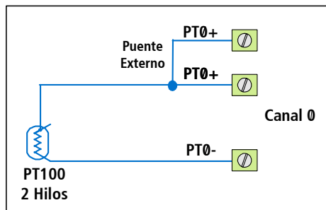
Figura 12 – Conexión PT100 2 Hilos
