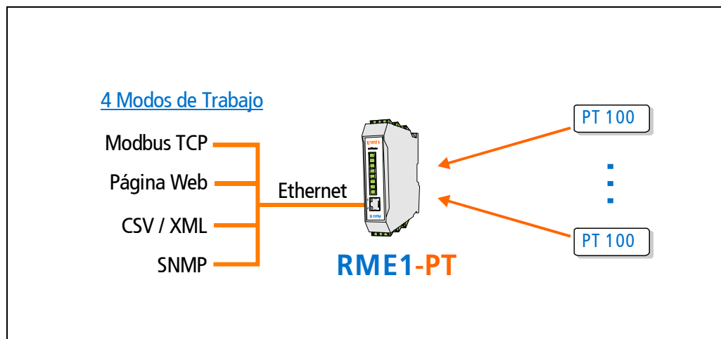
Figura 1 – Esquema General de uso.
