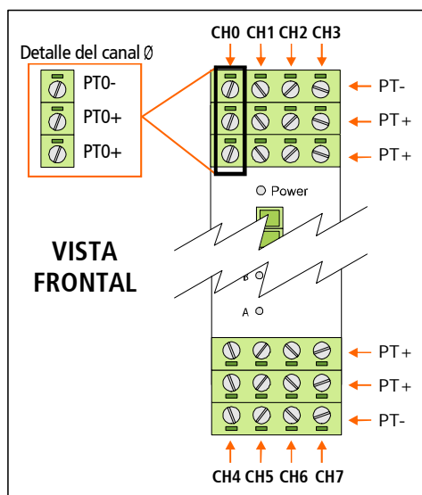
Figura 10 – Disposición de las entradas analógicas en cada canal del adquisidor RME1-PT
