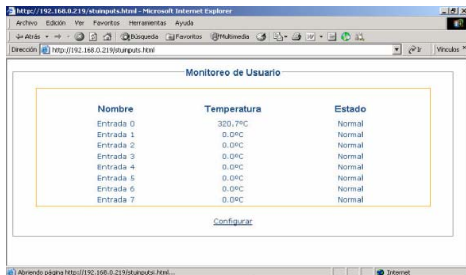
Figura 25 – Monitor de Usuario
