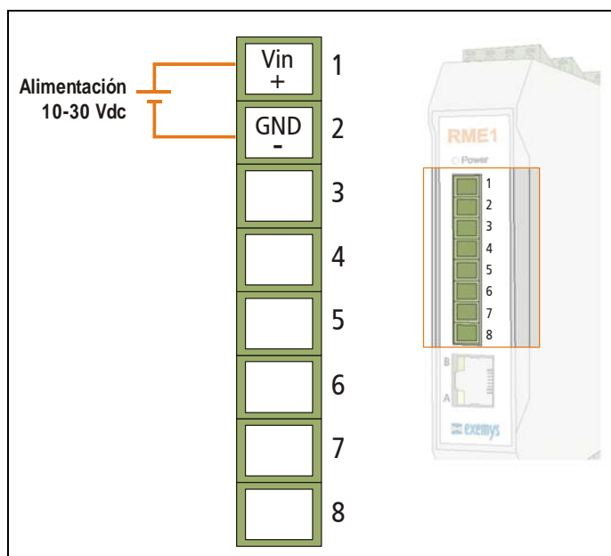
Figura 4 – Esquema de conexión de la alimentación
