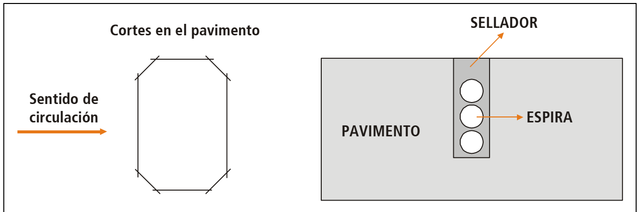
Figura 6 - Correcta instalación de una espira
