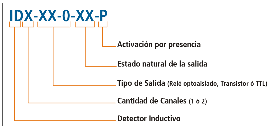
Figura 1 – Codificación
