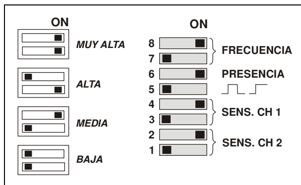
Figura 9 - Configuración de Fábrica
