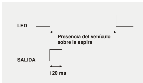
Figura 3 - Señal de salida por Pulso
