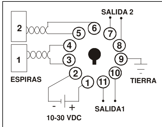
Figura 7 – Conexionado
