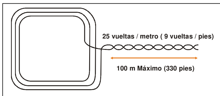
Figura 5 - Construcción de una espira
