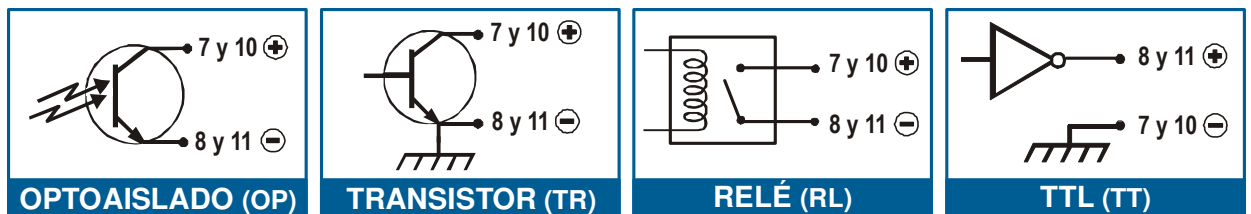
Figura 8 - Salidas Optoaisladas , Transistor, Rlé y Optoaisladas.
