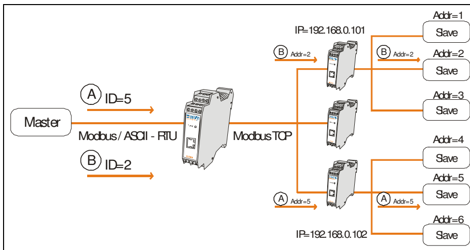
Figura 9 -Paso de mensajes a través de EGW1-MB MASTER
