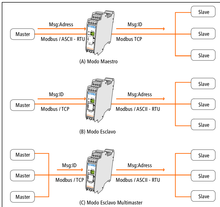
Figura 7 - Diagramas de Master, Slave y Slave-Multimaster
